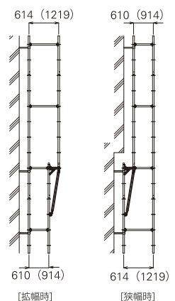
使用状態図
